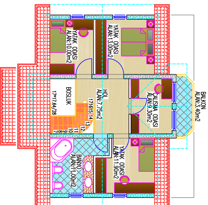
1.KAT PLANI 66.60 m 2 (1.ALTERNATIF)
